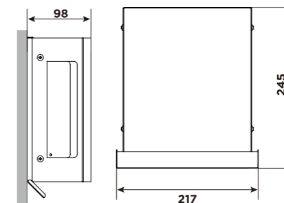
■フード寸法図
