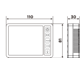
■リモコン寸法図
