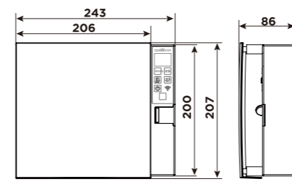
■本体寸法図
